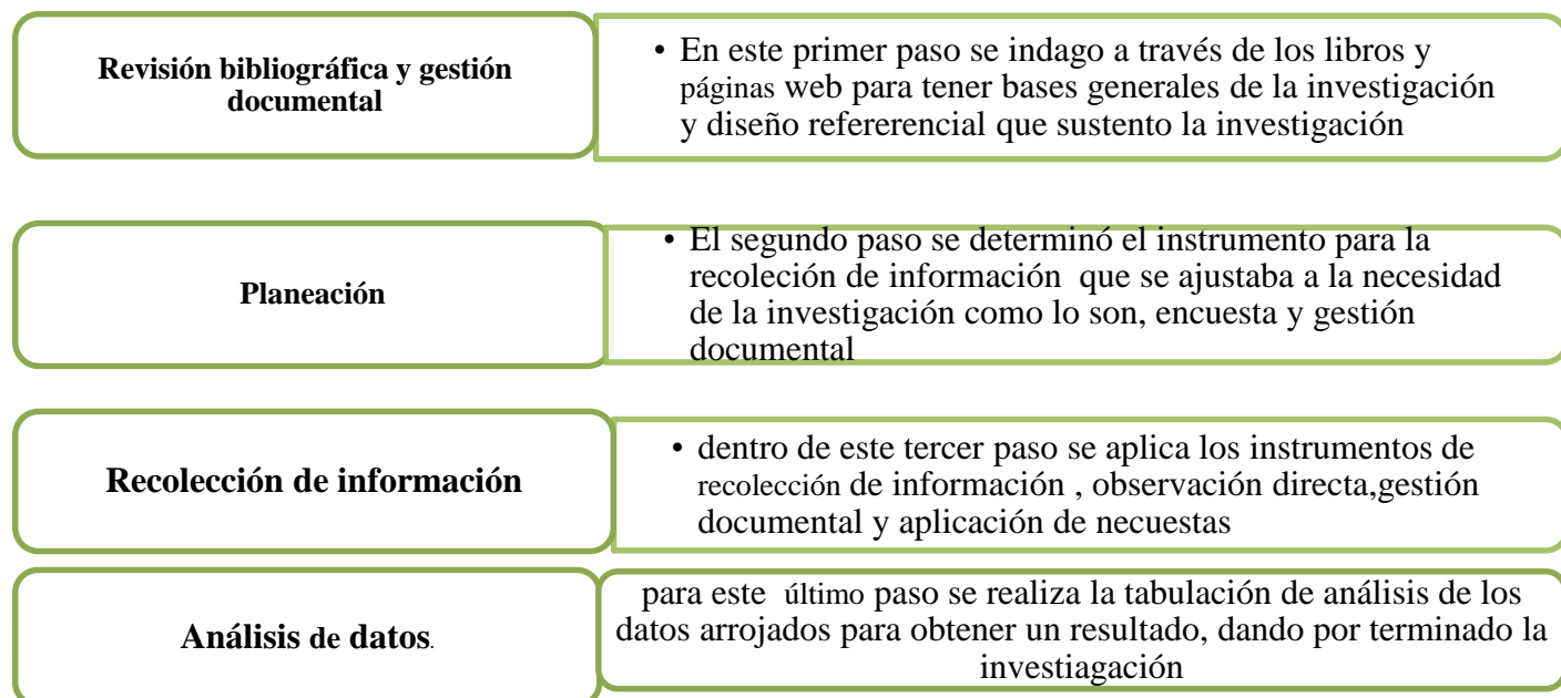
Gráfico 2. Procedimiento metodológico
