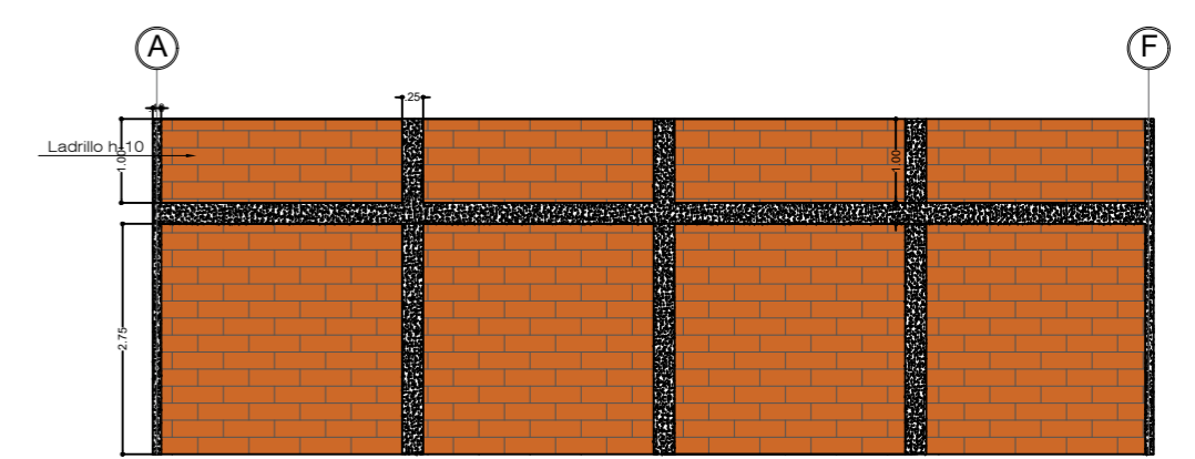
FACHADA POSTERIOR
